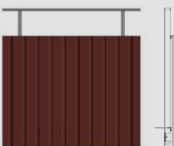
Täckning B med TRP-plåt
