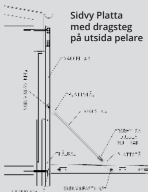
Dragsteg på utsida pelare
