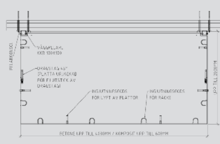
Dragsteg på utsida pelare
