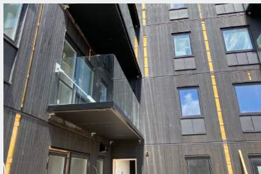
Kompositplattor med dragsteg och plattkantsavtäckning.
