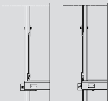
Frontvy Dragstag på insida/utsida pelare
