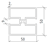
Alba ramprofil
